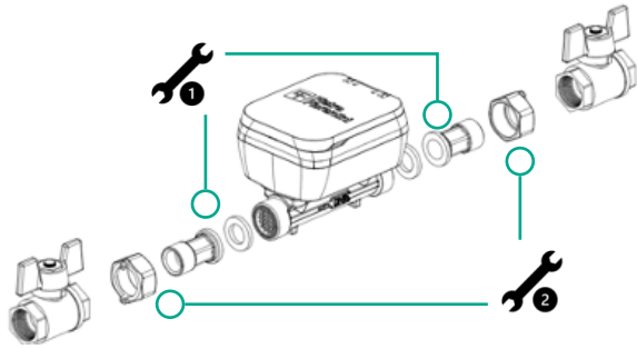
Fig. 1.6. meter joints
